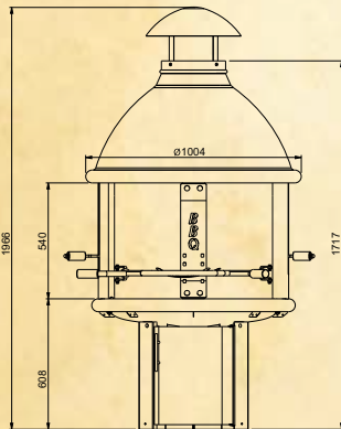
KOTAKEITTIÖ® BBQ MATALA MALLI
