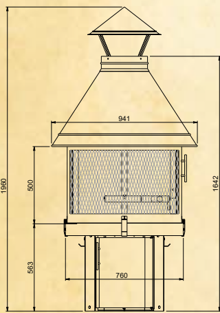
KOTAKEITTIÖ® CITY MATALA MALLI
