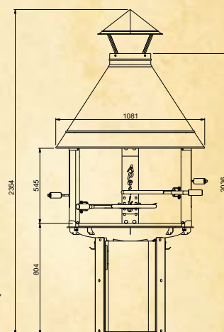
KOTAKEITTIÖ® APETIVO KORKEA MALLI
