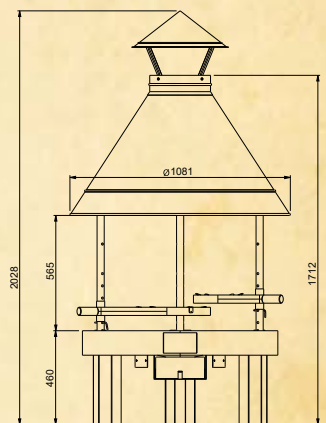
KOTAKEITTIÖ® 100 MATALA MALLI
