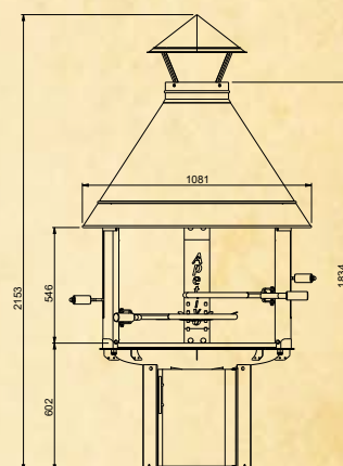
KOTAKEITTIÖ® APETIVO MATALA MALLI
