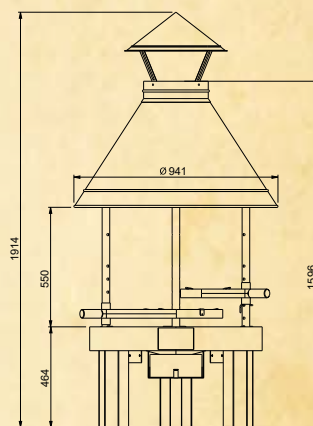
KOTAKEITTIÖ® 80 25V. JUHLAMALLI MATALA MALLI
