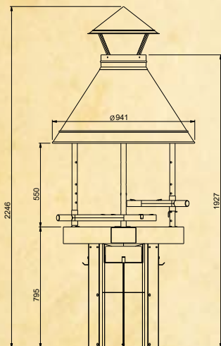
KOTAKEITTIÖ® 80 KORKEA MALLI
