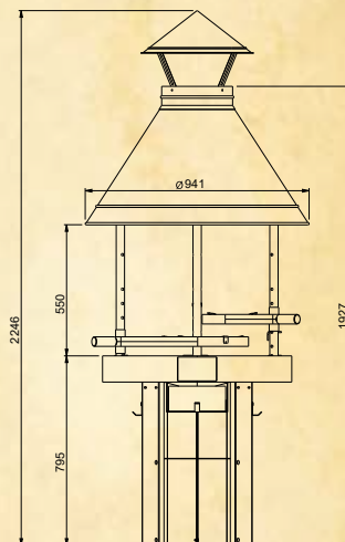
KOTAKEITTIÖ® 80 25V. JUHLAMALLI KORKEA MALLI
