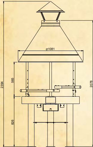
KOTAKEITTIÖ® HEAVY DUTY KORKEA MALLI
