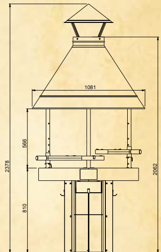
KOTAKEITTIÖ® 100 KORKEA MALLI
