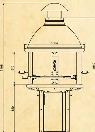
KOTAKEITTIÖ® BBQ KORKEA MALLI
